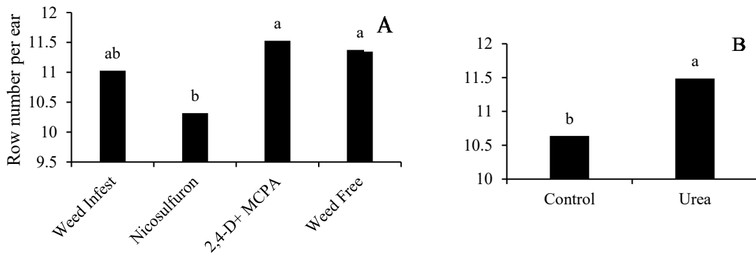
شکل ۳- اثرات اصلی روش کنترل علف‌هرز و کود بر تعداد ردیف در بلال ذرت. حروف مشابه نشان‌دهنده عدم اختلاف معنی‌دار در سطح پنج درصد احتمال است.
