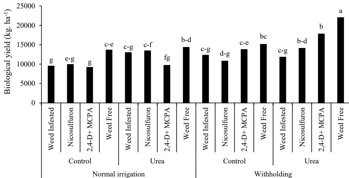
شکل ۴- تأثیر برهمکنش آبیاری، کود دهی و روش کنترل علف‌هرز بر عملکرد بیولوژیک ذرت. حروف مشابه نشان‌دهنده عدم اختلاف معنی‌دار در سطح پنج درصد احتمال است.
