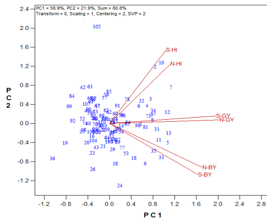
شکل ۶. نمایش برداری نمودار دووجهی نژادگانهای گندم در شرایط بدون تنش و تنش شوری Figure 6. Biplot vector view of wheat genotypes in non-stress and saline stress conditions
