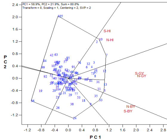
شکل ۵. نمایش چندضلعی نمودار دووجهی نژادگانهای گندم در شرایط بدون تنش و تنش شوری Figure 5. Biplot polygon view of wheat genotypes in non-stress and saline stress conditions
