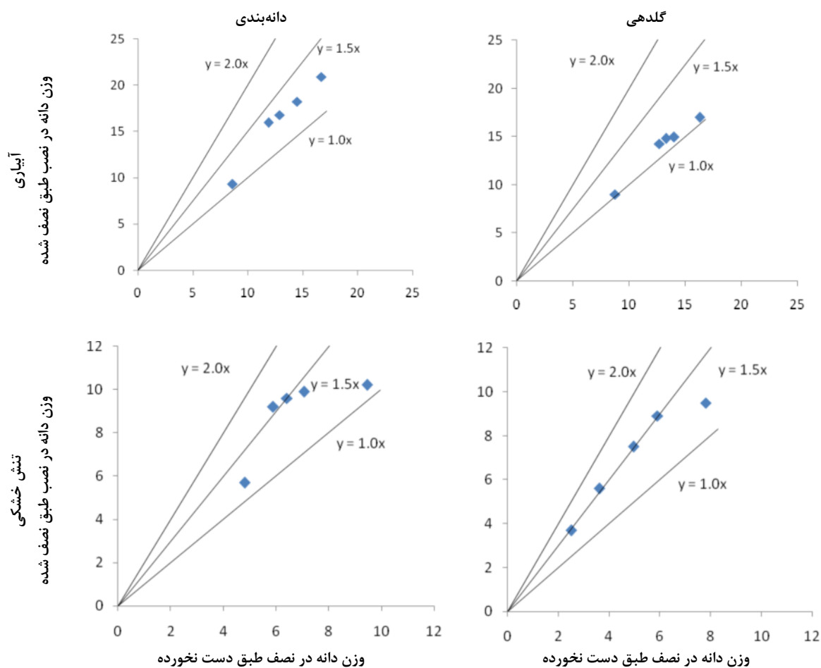
شکل ۱- متوسط وزن دانه‌های نصف طبق در طبق‌های نصف شده در مقایسه با طبق‌های دست نخورده در رقم آذرگل آفتابگردان در شرایط آبیاری و تنش خشکی. در هر شکل نقاط از راست به چپ به ترتیب نشان‌دهنده میزان ۰٪، ۲۵٪، ۵۰٪، ۷۵٪ و ۱۰۰٪ برگ‌زدایی می‌باشد. خط Y=1.0X نشان‌دهنده محدودیت کامل مخزن، خط Y=1.5X نشان‌دهنده محدودیت عملکرد ناشی از هر دو عامل منبع و مخزن، خط Y=2.0X نشان‌دهنده محدودیت کامل منبع است. هر نقطه در هر شکل میانگین سه تکرار است.
