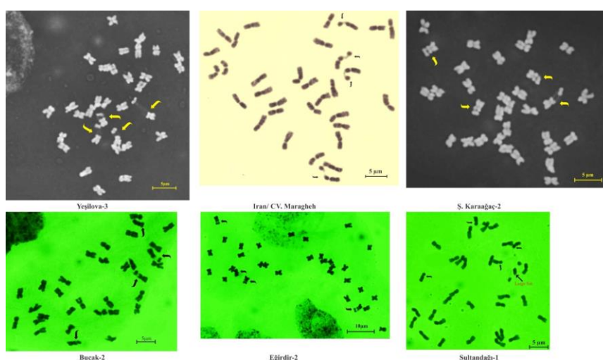
شکل ۲. یاخته‌های سوماتیک جمعیت‌های یونجه ( Medicago sativa L.) که با کلون افزونش شدند و 2n=4x=32 کروموزوم را نشان می‌دهند. کروموزوم‌های ماهواره‌دار با فلش‌ها نشان داده شده است. فلش نازک در جمعیت Sultandağı-1 ماهواره یا ماهواره بزرگ را نشان می‌دهد.
