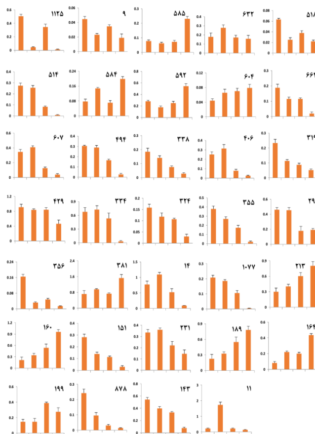
شکل ۳. مقایسه میانگین درصد حجمی لکه‌های پروتئینی مختلف با تفاوت معنی‌دار (گزینش‌شده) در هر نمودار (به‌ترتیب از سمت چپ به راست، متحمل (سرداری) شاهد - متحمل ۱۲- بار - حساس (قدس) شاهد - حساس ۱۲- بار)
