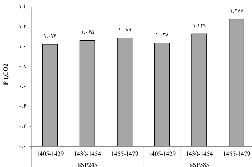
شکل ۴. شبیه‌سازی اثر دی‌اکسیدکربن بر عملکرد گندم تحت دو سناریوی SSP245 و SSP585.
