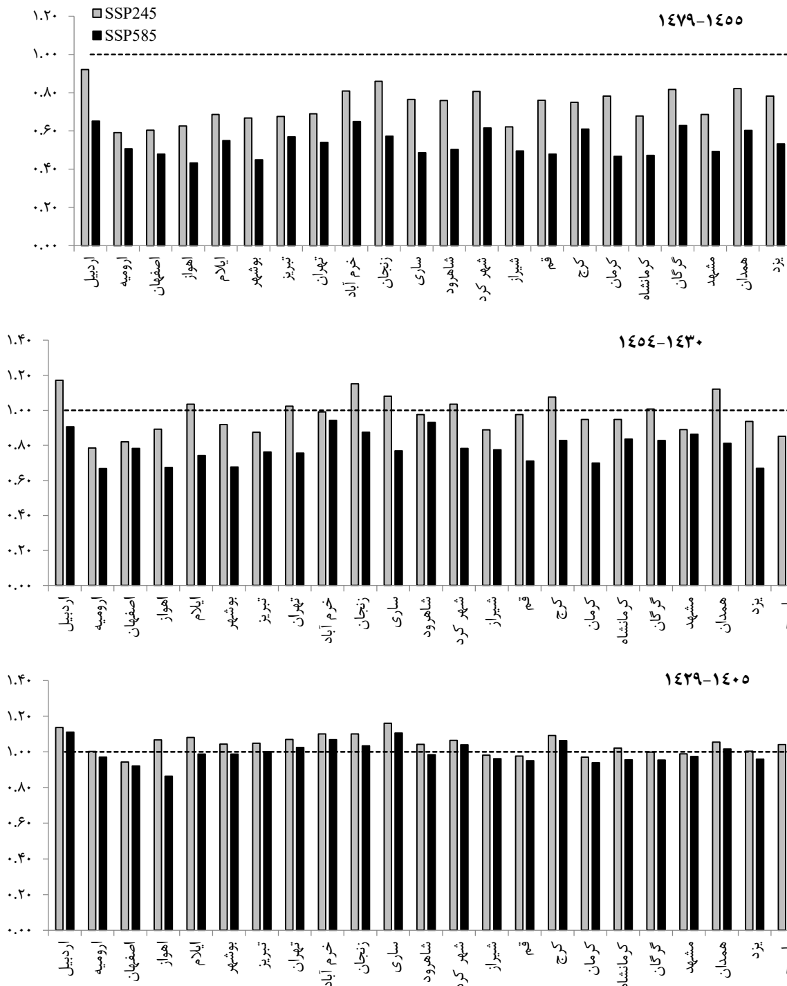
شکل ۵. اثرات تلفیقی (تغییر اقلیم، دی‌اکسید کربن و پیشرفت فناوری) بر عملکرد گندم در سناریوهای اقلیمی و دوره‌های زمانی مختلف. Figure 5. Integrated effects (climate change, CO 2 and technological advancement) on wheat yield under different climate scenarios and time periods.
