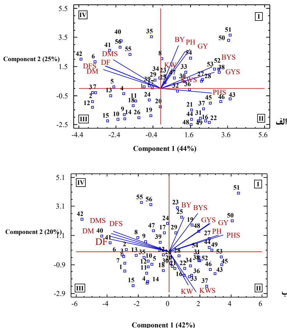
شکل ۲. نمودار بای پلات دو مولفه اصلی برای میانگین صفات مورد ارزیابی در ژنوتیپ‌های جو زراعی در سال زراعی ۱۳۹۹-۱۳۹۸ (الف) و ۱۳۹۹-۱۴۰۰ (ب) در ایستگاه یزد (GY: عملکرد دانه، BY: عملکرد بیولوژیکی، PH: ارتفاع بوته، DS: روز تا ظهور سنبله، DF: روز تا گلدهی، DM: روز تا رسیدن و KW: وزن هزار دانه، پسوند S به معنای شرایط تنش می‌باشد).
