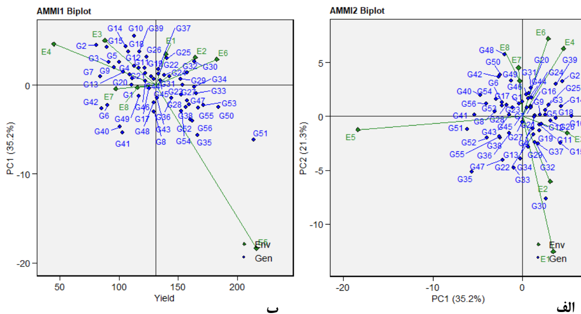
شکل ۴. نمودار AMMI2 بر پایه دو مؤلفه اصلی اول (الف) و AMMI1 بر پایه میانگین عملکرد دانه و مؤلفه اصلی اول (ب) و در ژنوتیپ‌های جو زراعی در دو شرایط تنش خشکی و نرمال در دو ایستگاه تحقیقاتی استان یزد و استان سیستان (زهک) و دو سال زراعی.
